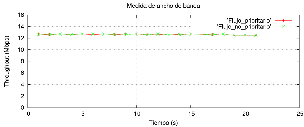
Figura 6.6: 2 flujos, qdisc sin prioridad, WMM desactivado
