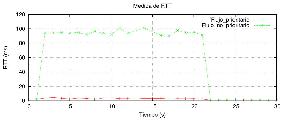
Figura 6.8: RTT de 2 flujos, qdisc sin prioridad, WMM parámetros por defecto
