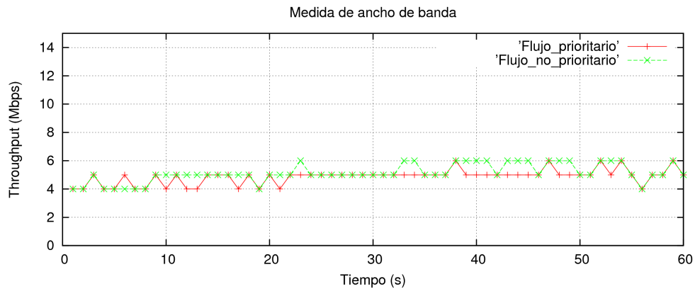
Figura 9.6: Configuración sin qdisc ni 802.11e.
