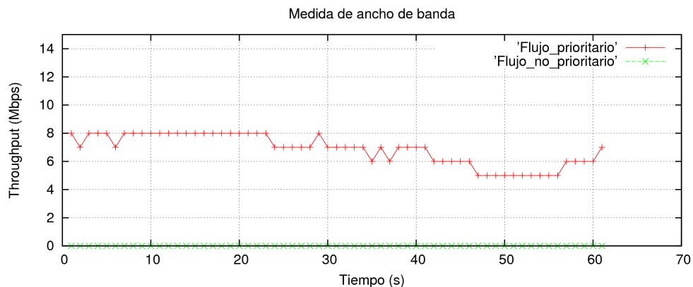
Figura 9.3: Bandwidth obtenido con la configuración seleccionada
