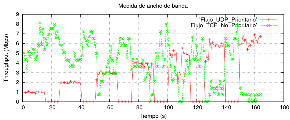
Figura 9.12: Throughput flujo TCP y UDP sin QoS
