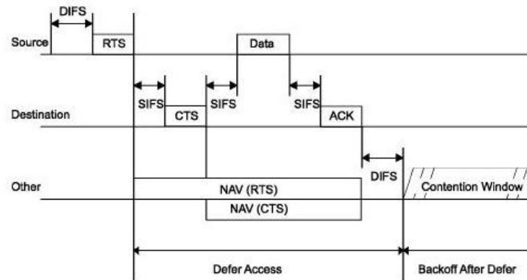
Figura A.5: Procedimiento RTS/CTS
