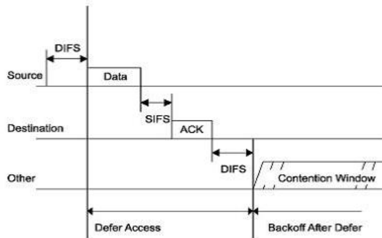
Figura A.6: Procedimiento ACK
