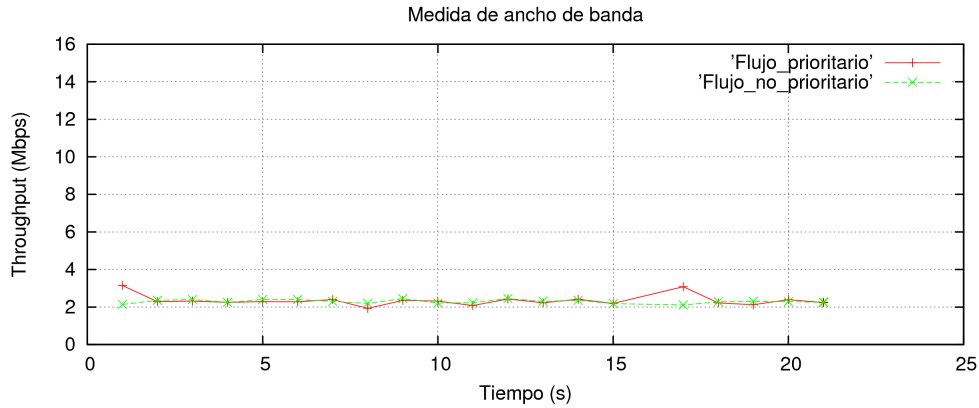
Figura 6.9: 2 flujos, qdisc sin prioridad, clase AC_BK de 802.11e degradada
