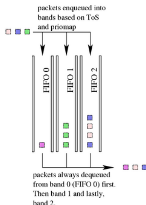
Figura E.1: Pfifo fast
