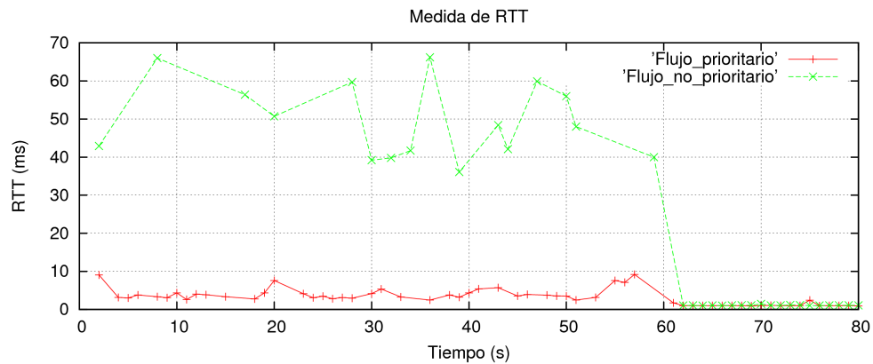
Figura 9.2: RTT obtenido con la configuración seleccionada
