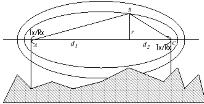
Figura 7.1: Elipsoides de Fresnel
