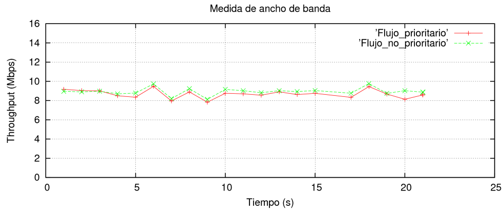
Figura 6.5: WMM, AC_BK degradado pero txop = 8192
