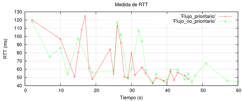
Figura 9.7: Configuración sin qdisc ni 802.11e.
