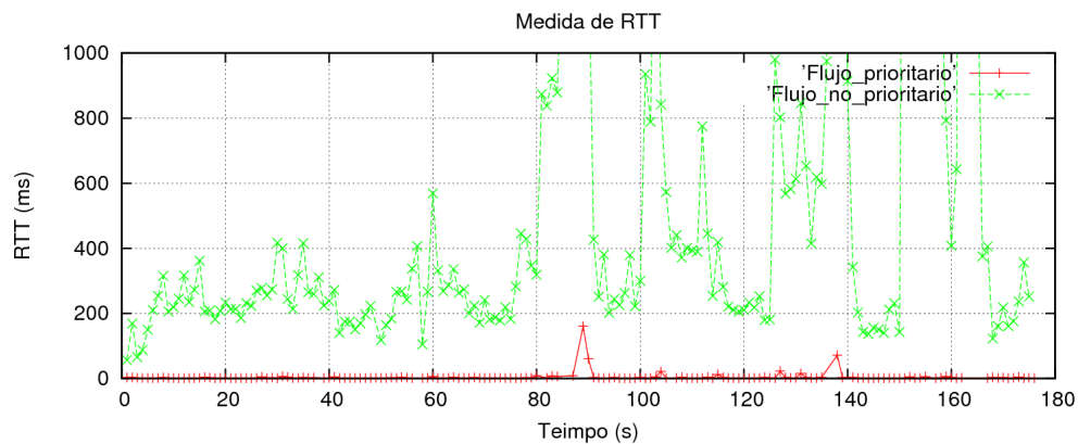
Figura 9.11: Retardo flujo TCP y UDP
