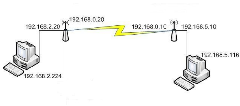
Figura 5.1: Arquitectura de pruebas de laboratorio
