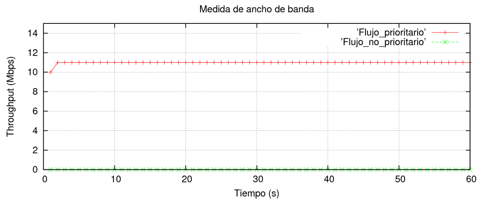
Figura 9.1: Bandwidth obtenido con la configuración seleccionada
