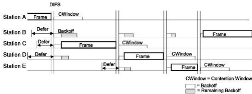
Figura A.4: Procedimiento Backoff .
