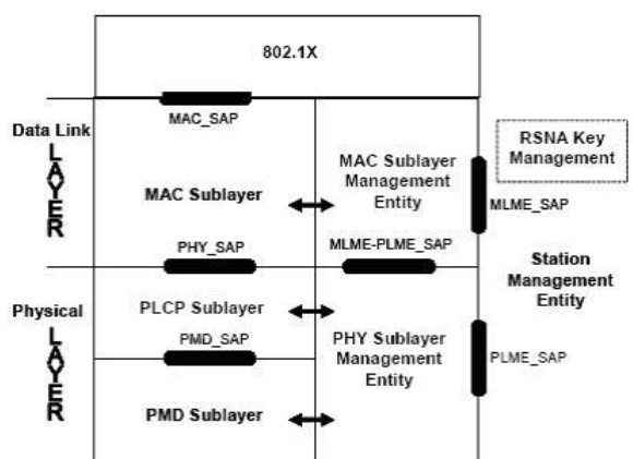
Figura A.1: Modelo de referencia.
