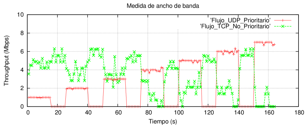
Figura 9.10: Throughput flujo TCP y UDP
