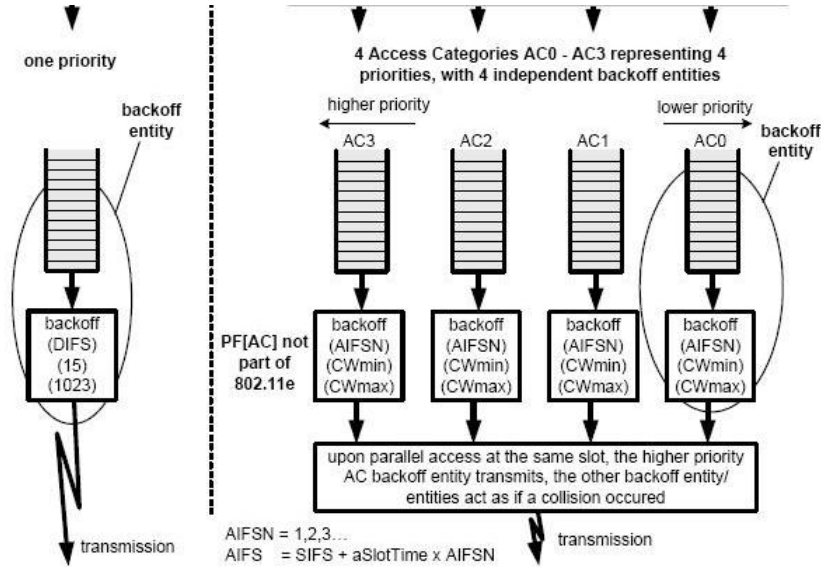
Figura 2.1: Comparación del modo de funcionamiento en 802.11 y 802.11e [?]
