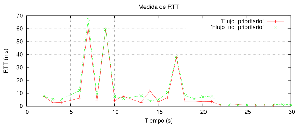
Figura 6.15: 2 flujos, qdisc con prioridad, WMM deshabilitado
