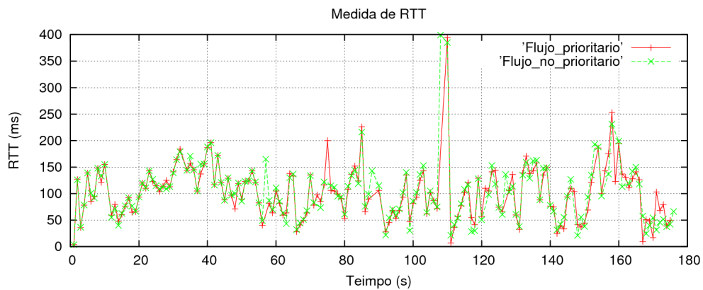
Figura 9.13: Retardo para TCP y UDP sin QoS
