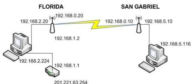
Figura 8.6: Diagrama de topología
