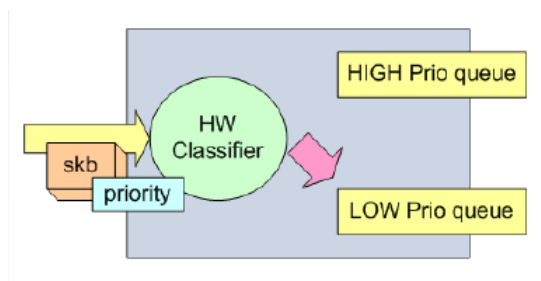
Figura 6.10: 2 colas en hardware [?]
