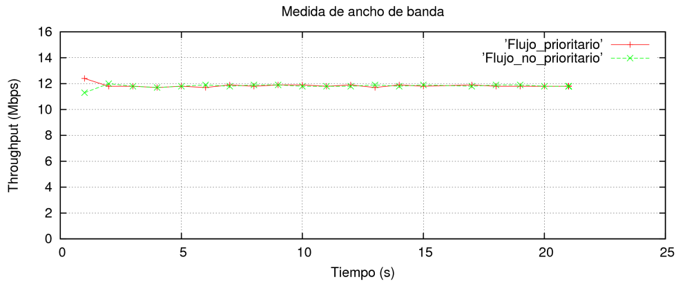
Figura 6.7: 2 flujos, qdisc sin prioridad, WMM parámetros por defecto
