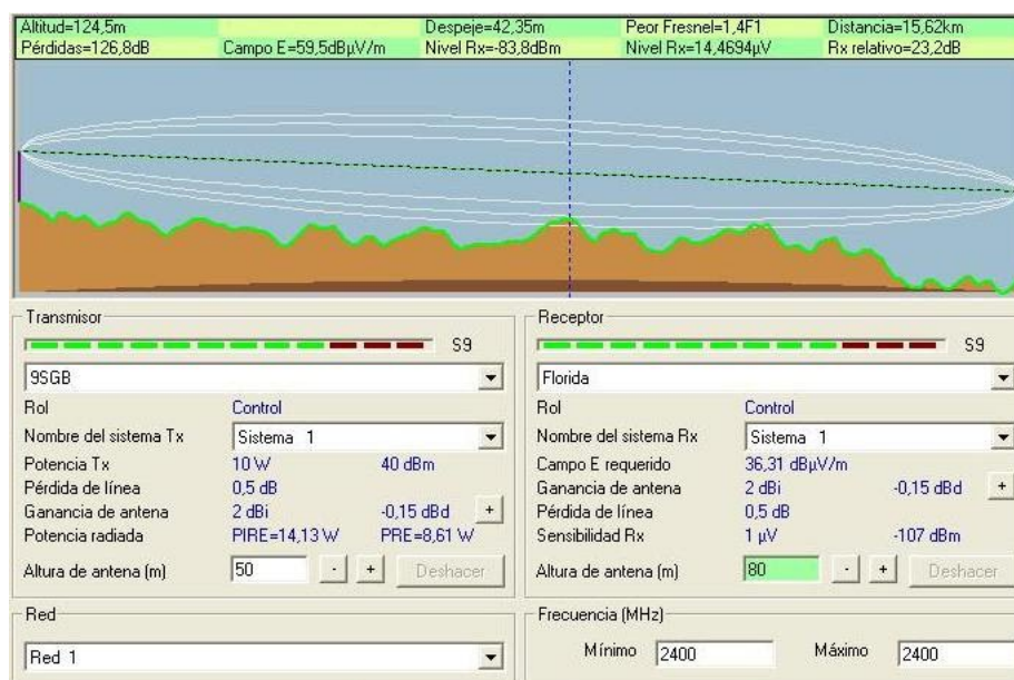
Figura 8.2: Análisis de Fresnel para 2.4 GHz
