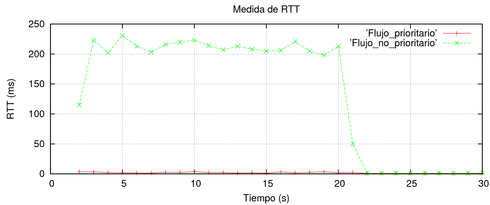
Figura 6.14: 2 flujos, qdisc con prioridad, WMM por defecto
