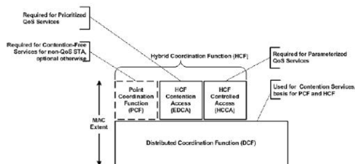
Figura A.2: Arquitectura de la subcapa MAC
