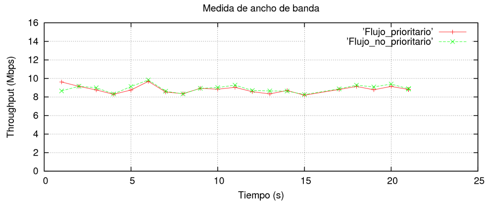
Figura 6.11: 2 flujos, qdisc sin prioridad, clase AC_BK de 802.11e degradada con txop de AC_BK = 8192
