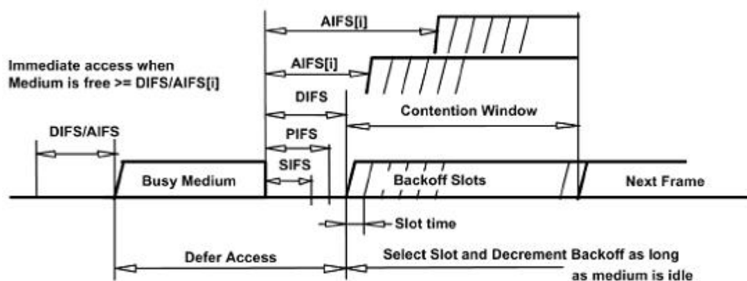
Figura A.3: Relación de distintos IFS.
