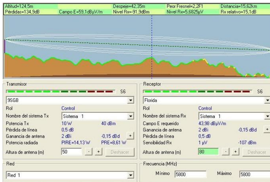
Figura 8.3: Análisis de Fresnel para 5.8 GHz
