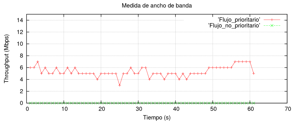
Figura 9.5: Qdisc sin 802.11e.
