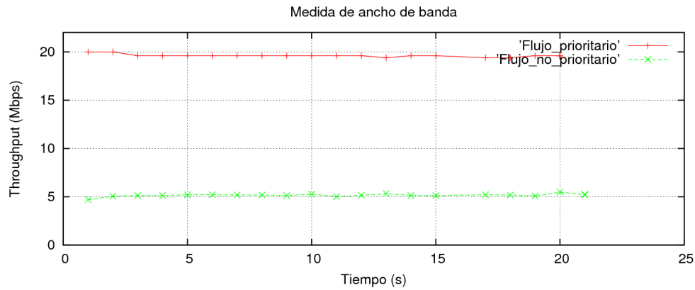
Figura 6.13: 2 flujos, qdisc con prioridad, WMM por defecto
