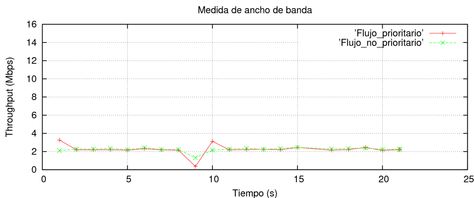
Figura 6.12: 2 flujos, qdisc sin prioridad, clase AC_BK de 802.11e degradada con txop de AC_VO = 8192
